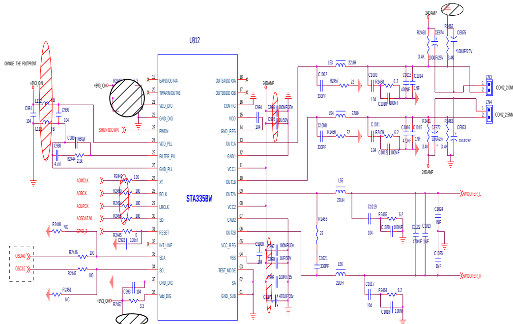
图 12 功放 STA335BW 外围电路图
