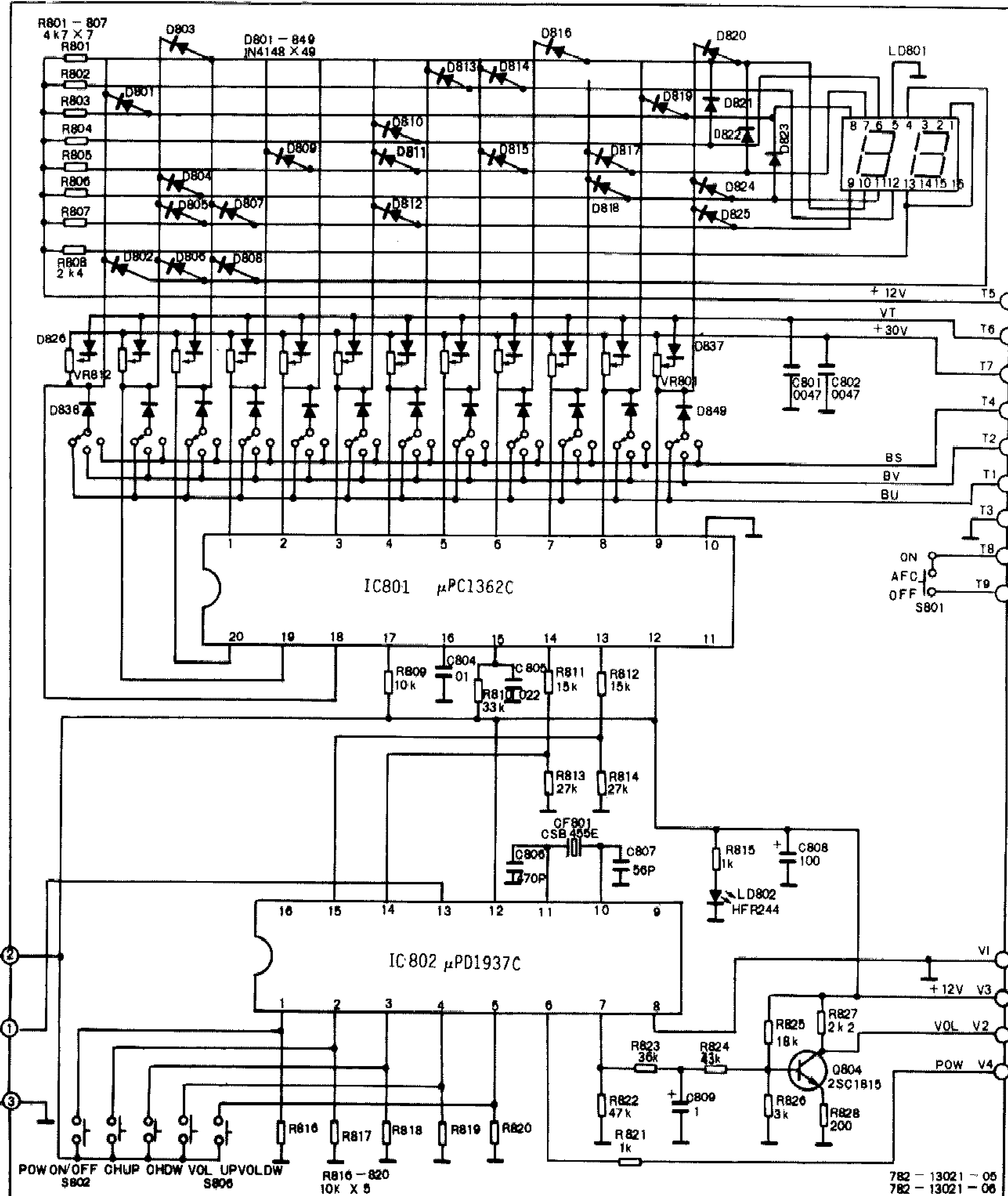
通道选择和遥控接收板
