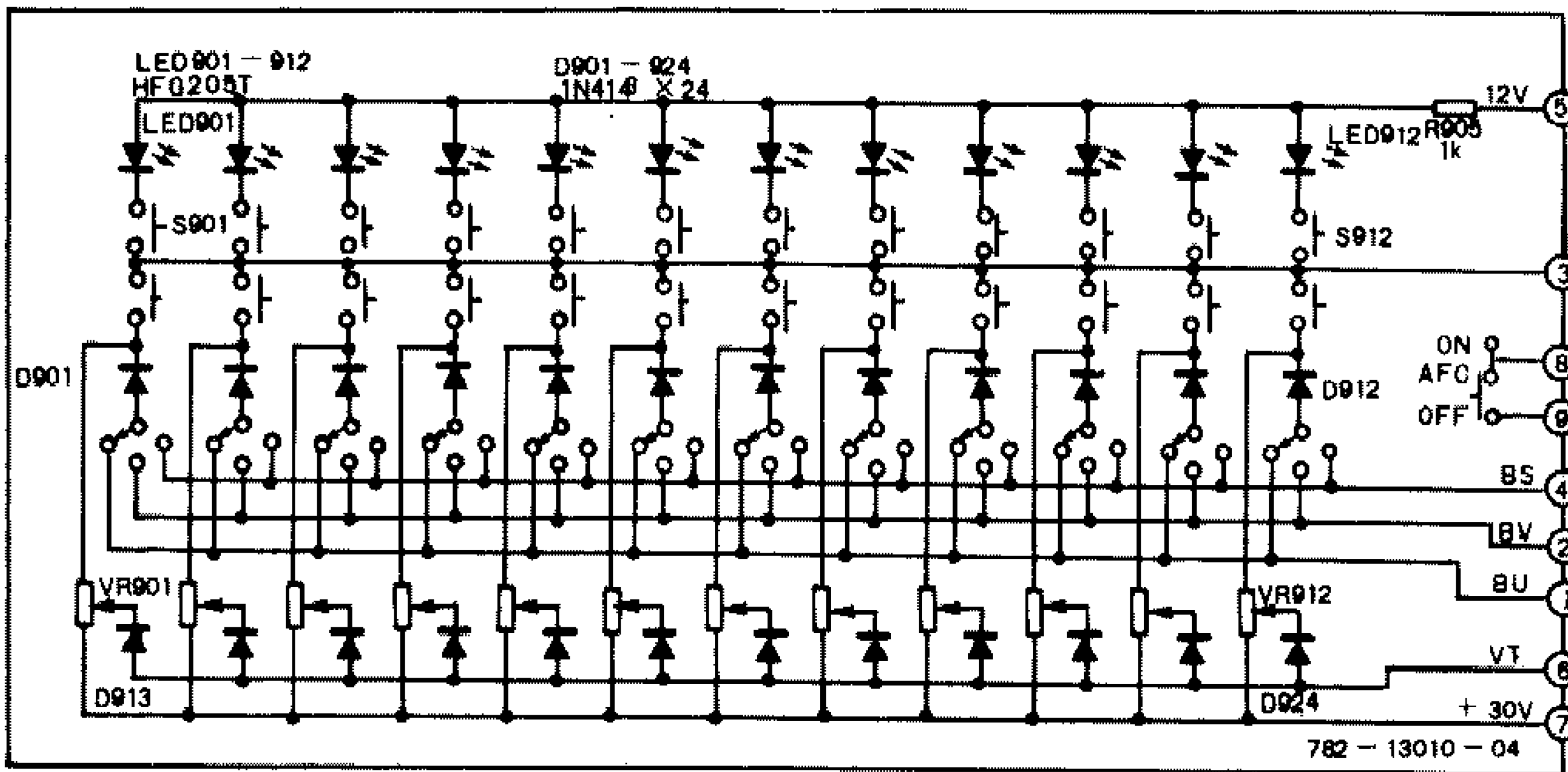
遥控发射板
