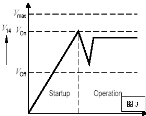
图 2 为启动电路；图 3 为启动电压过程图，图中 V_{on} 和 V_{off} 为供电比较器的上门限和下门限，Startup 启动，Operation 正常工作
