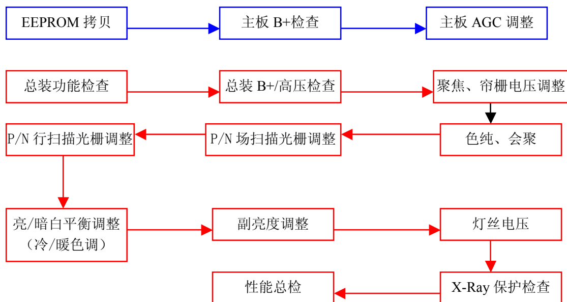
图1 调校流程图
