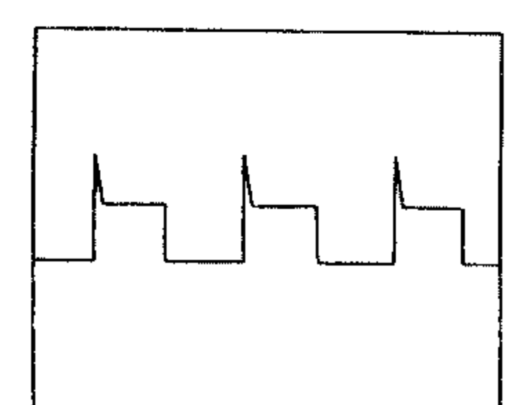
⑨ 80Vp-p H
