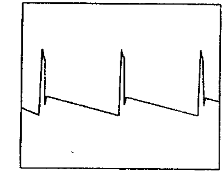
⑬ 56Vp-p V
