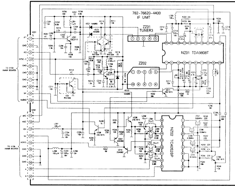
中放板
